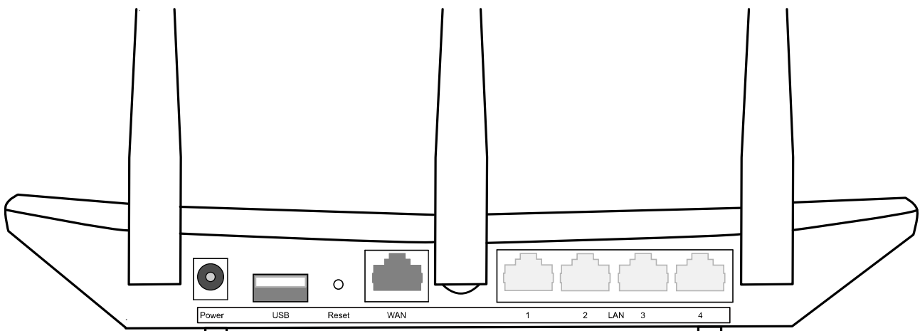
图 2-2 TL-WVR450A后面板示意图
