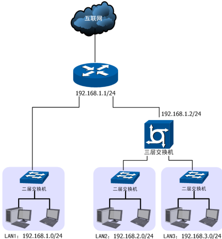
图 4-55 静态路由功能组网应用
