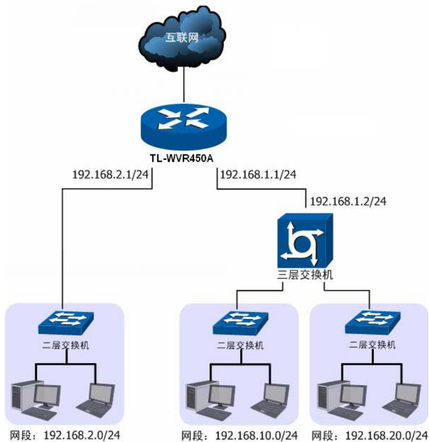
图 4-45 NAPT功能组网应用
