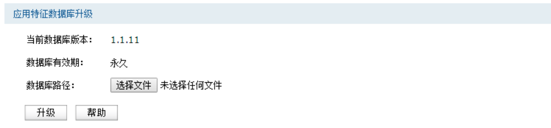
图 4-74 策略库升级界面
